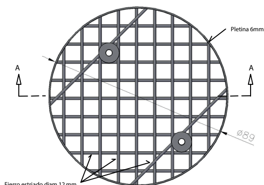
VISTA PLANTA
