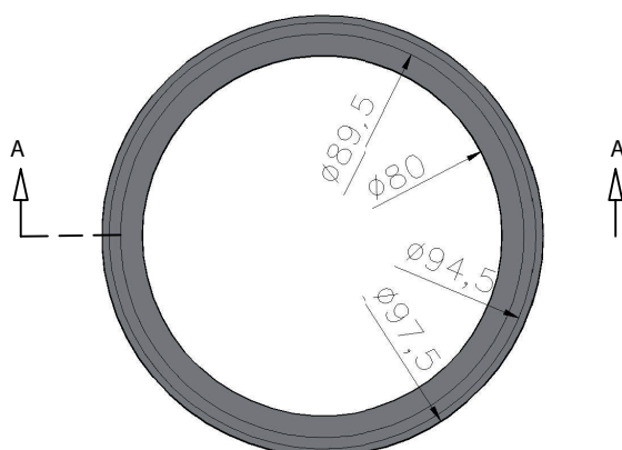
VISTA PLANTA
