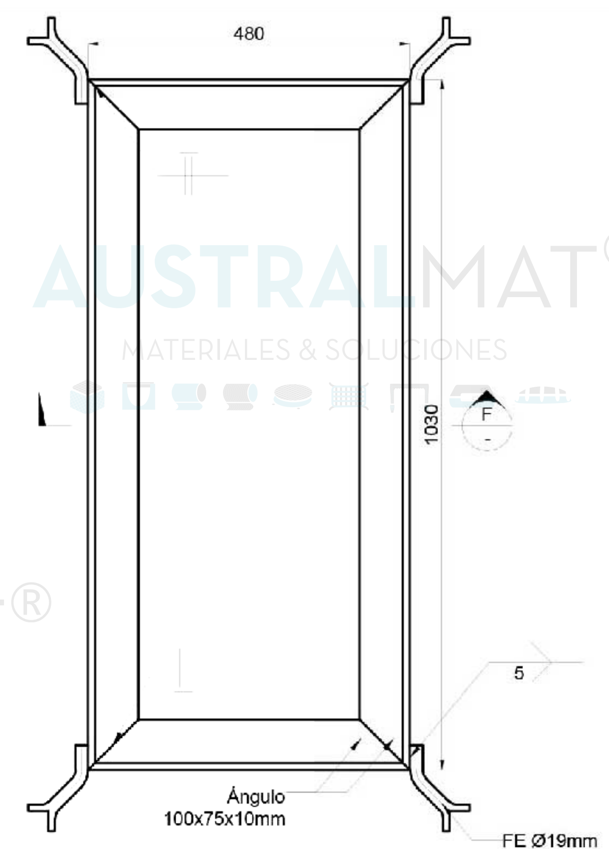
MARCO DE ÁNGULOS REJILLA TIPO 45-9-R
