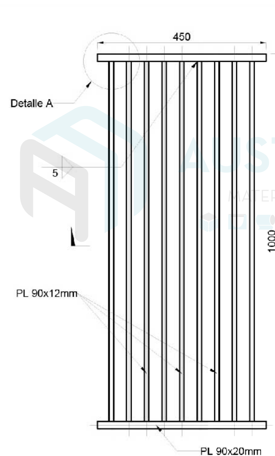
REJILLA TIPO 45-9-R
